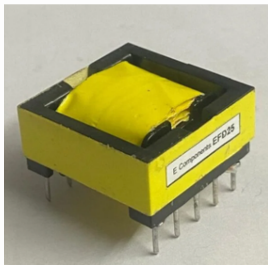
EFD 25x13x7 10P "H"
