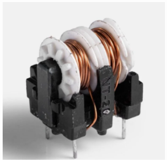
UT20 4P "V"
