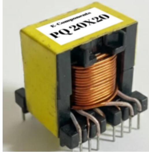
PQ20x20 14P "V"
